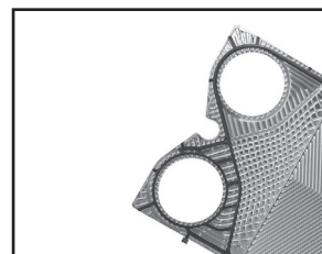
Joints d'échangeur à plaque
